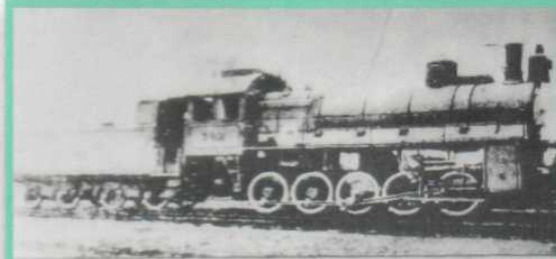
Паровоз серії „Е” побудований 1912 р. заводами Росії Вага 80,6 тонн. Колесникова решітка 4,46 м 2 , тиск пари 12 атмосфер ( в депо Гречани працювали з 1938 р.)
