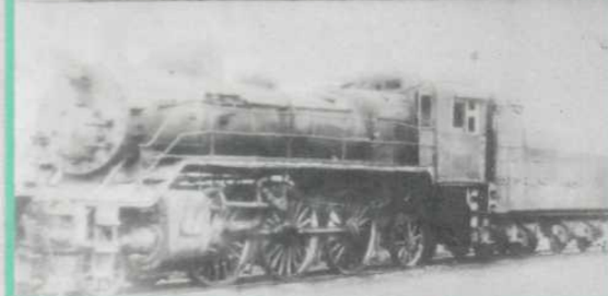
Паровоз серії „С” типу 1-3-1, побудований в 1910 р. Сормовським заводом Вага 75,8 тонн. Колесникова решітка 4,46 м 2 , тиск пари 12 атмосфер ( в депо Гречани працювали з 1938 р.)
