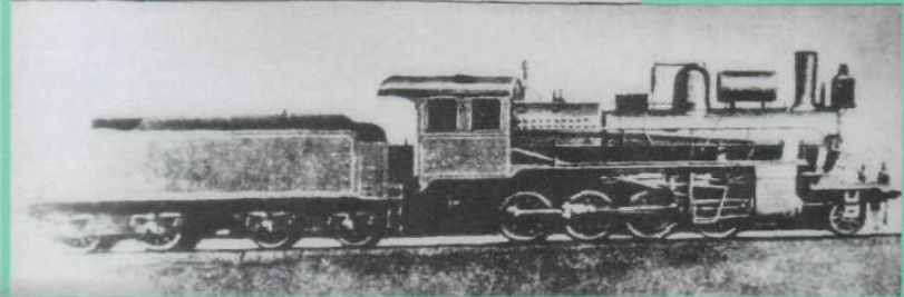
Паровоз серії „Щ” типу 1-0-4, побудований 1910-1911 рр. Сормовським заводом Вага 77 тонн. Колесникова решітка 2,8 м 2 , тиск пари 14 атмосфер ( в депо Гречани працювали в грузовому русі 1935-1939 рр.)
