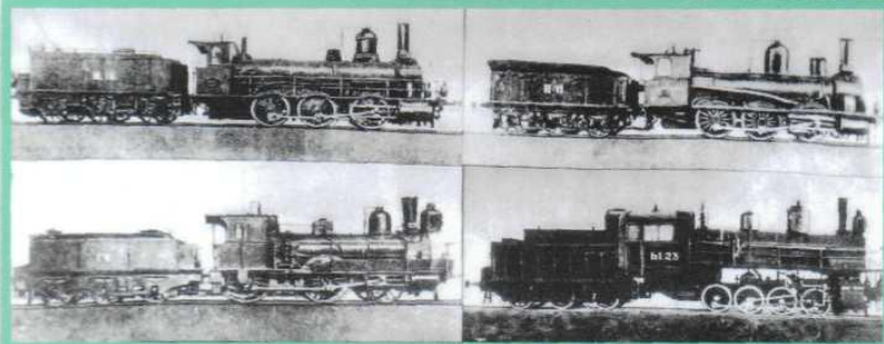
Паровоз серії „М” типу 0-3-0, побудовані 1872-1878 рр. Мальянським заводом, вага 39 тонн. Колесникова решітка 1,5 м 2 , тиск пари 9 атмосфер ( в депо Гречани працювали в 1915 році).
