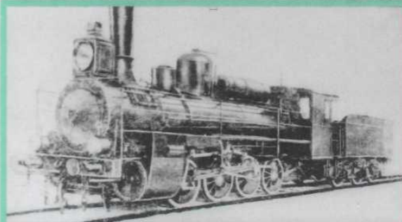
Паровоз серії „ОВ” типу 0-4-0, побудований 1912 р. Луганським заводом Вага 53,2 тонн. Колесникова решітка 1,85 м 2 , тиск пари 12 атмосфер ( в депо Гречани працювали в 1930-1935 рр.)
